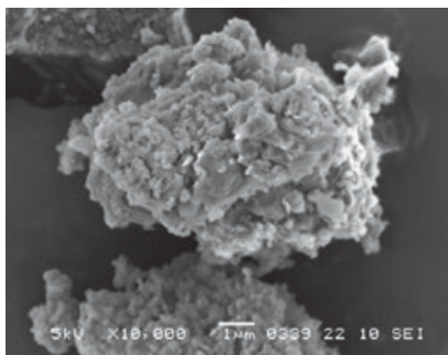
写真4 フロン分解物で融けたアスベスト
