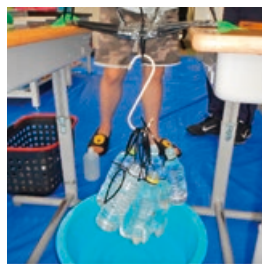
図2 ストローブリッジの強さの評価方法
